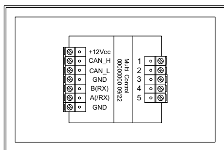
Aizmugurējais skats: savienojuma spaiļes
