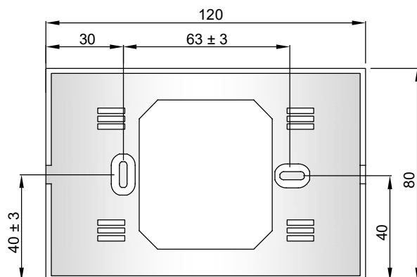
Instalācijas plāksne elektrības kārbai 502 vai apaļai
