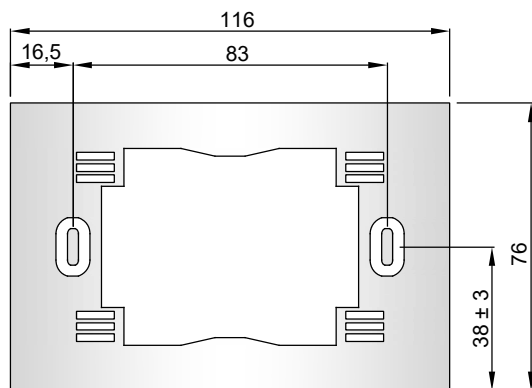
Elektrības kārbas 503 uzstādīšanas plāksne
